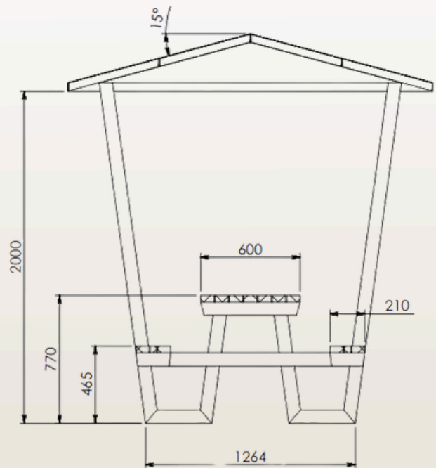
COUPE A-A
